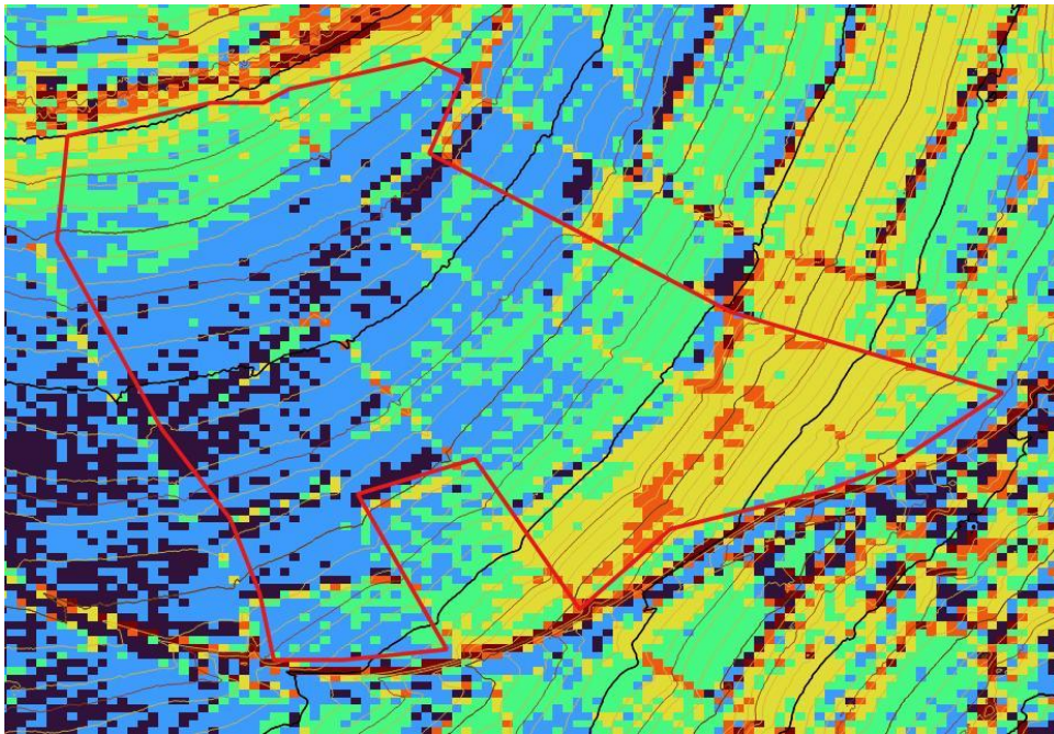
Abbildung 2: Hangneigung (dunkelblau: < 3^\circ , hellblau: < 5^\circ , grün: < 7^\circ , gelb: < 10^\circ , orange: < 15^\circ , rot: \geq 15^\circ ) sowie Höhenlinien (schwarz: 5m, braun: 2,5m) und Grenzen des Solarparks. Die Darstellung basiert auf eigenen Berechnungen, aufbauend auf dem DGM1. Datenquelle: Landesamt für Digitalisierung, Breitband (Bayern)
